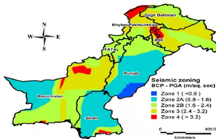
Figure-8 Seismic Zone Map
